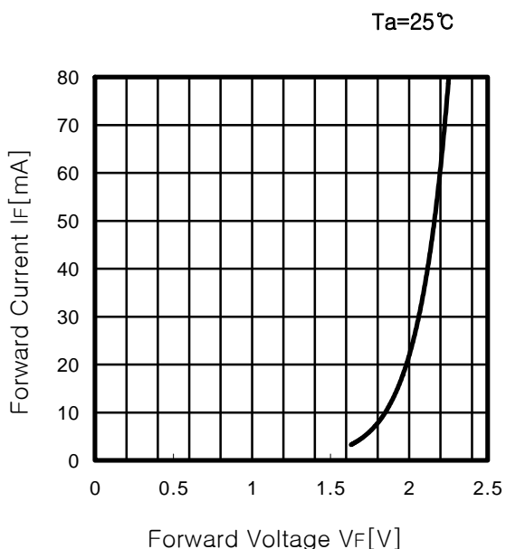
Fig.1 I_F - V_F
